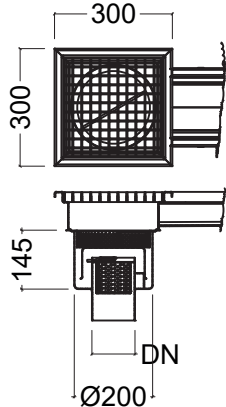
ÇIKIŞ KUTUSU, ALTTAN ÇIKIŞLI
