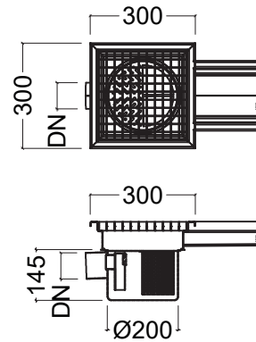
ÇIKIŞ KUTUSU, YATAY ÇIKIŞLI
